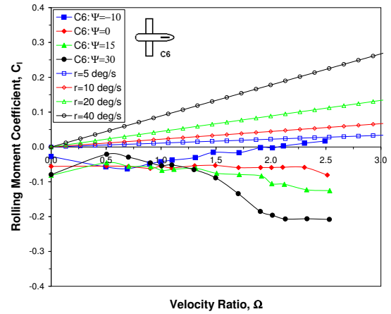
(d) Rolling moment results for C6
