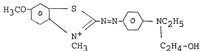
C.I. Maxilon Blue GRL
