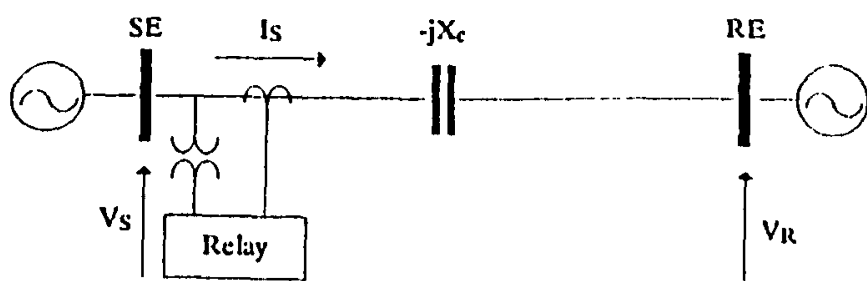
Fig 1:SYSTEM CONFIGURATION
