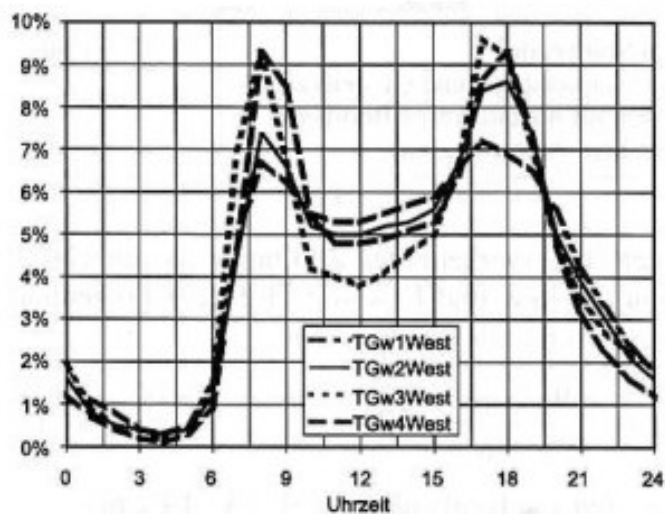
Abb. 3.3-1: Tagesganglinien der Verkehrsstärke (Quelle: HBS 2001)
