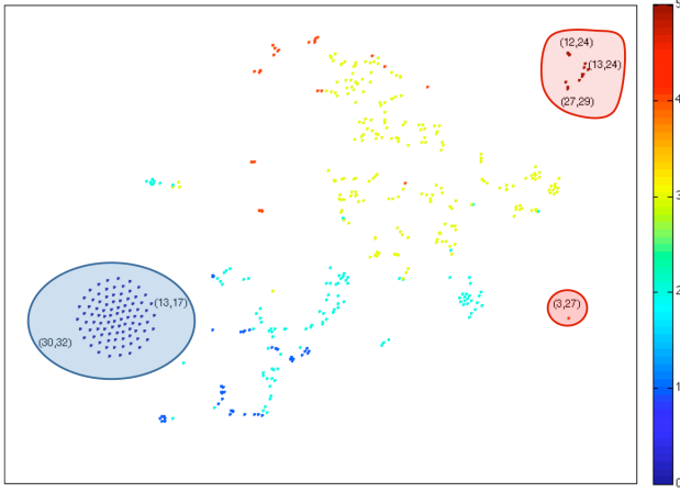
Figure 7. Visualizing failure rates of AV pairs using Multidimensional Scaling
