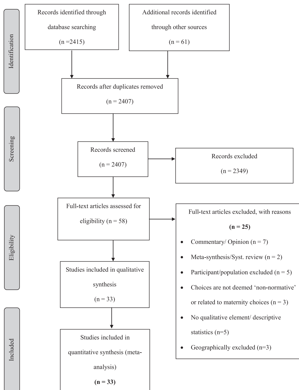
Fig. 1. Prisma diagram.
