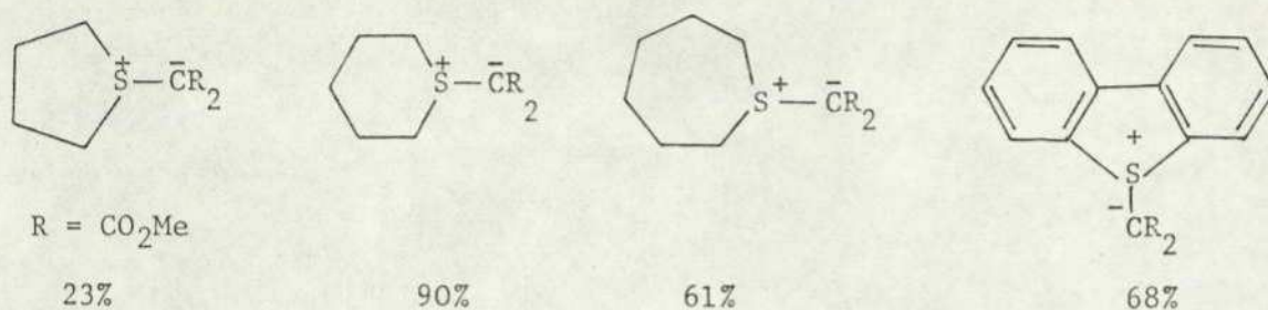
Scheme 14.
