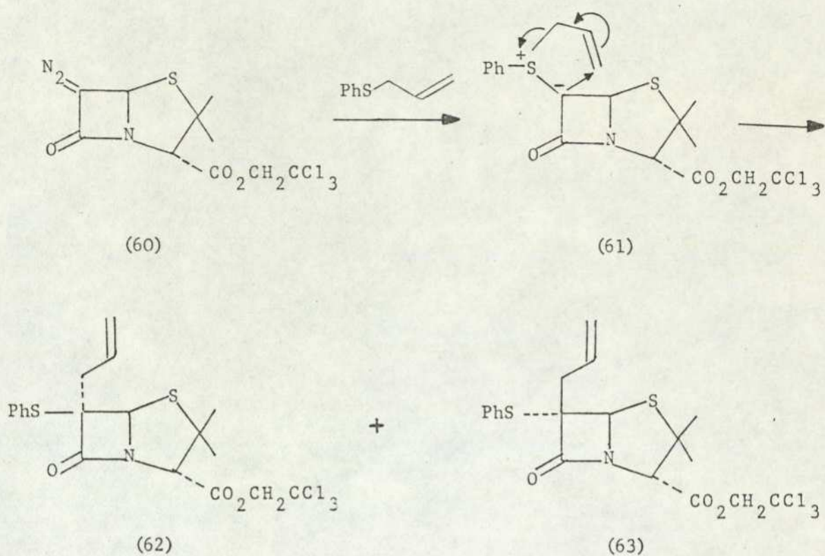
Scheme 16.
