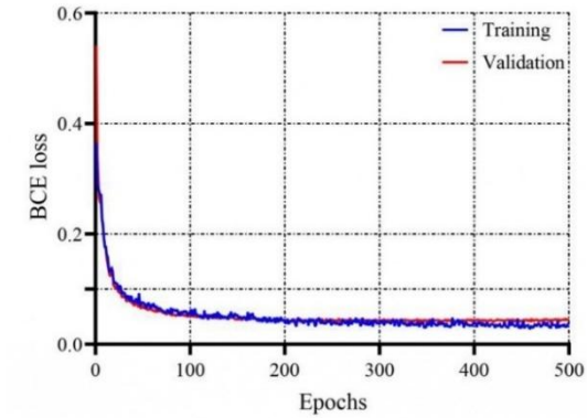
(d) Stage 2: CNN512 for simply supported dataset
