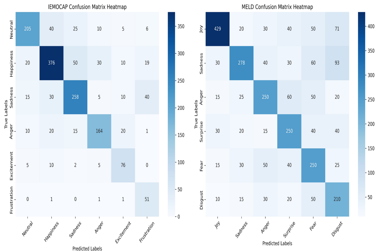
Fig. 8. Confusion matrix.
