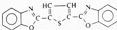
Benzoxazolyl
