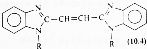
Benzimidazolyl
