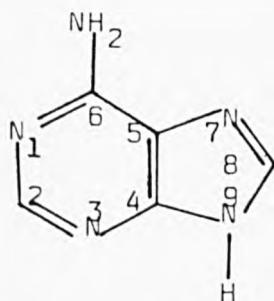
(d) Adenine
