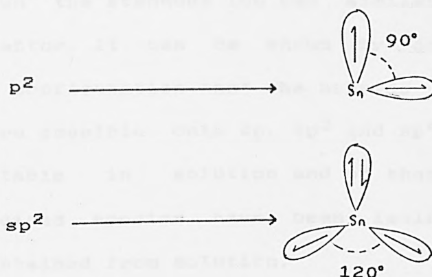
Fig.1.7. Sn Hybridisation in SnX_2
