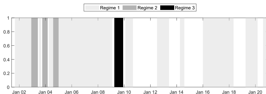
(d) Robustness 4
