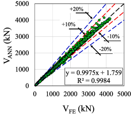
(a) ANN
