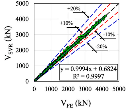
(b) SVR
