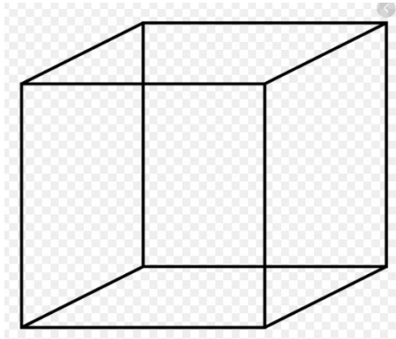
Fig. 4 Necker Cube
