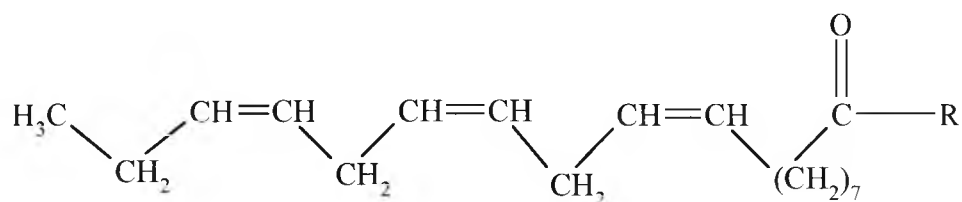
Linolenate.
