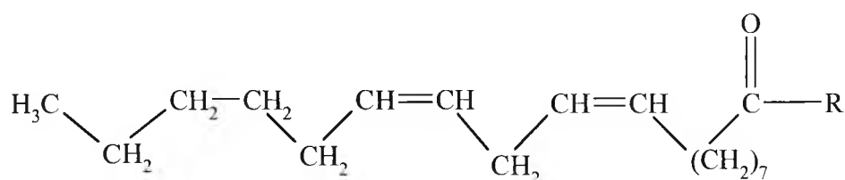
Linoleate.
