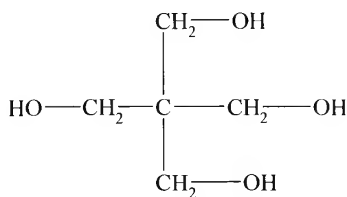
pentaerythritol
