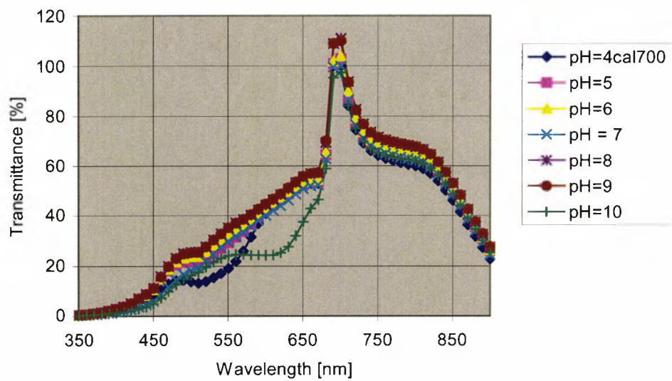
Fig.8.7: Universal pH Indicator Spectra.
