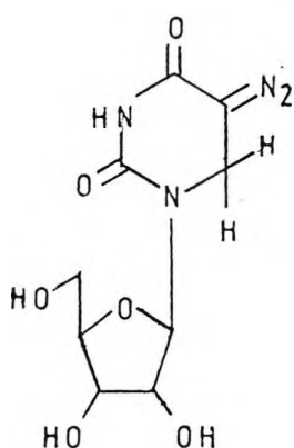
m/z 313 (9.30)
