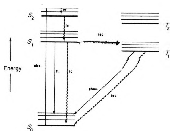
Fig. 1.7 Jablonski Diagram
