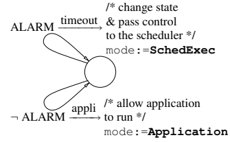
Fig. 6 Timeout automaton
