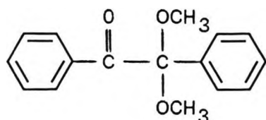
Irgacure 651
