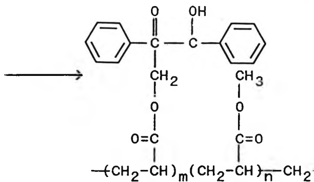
MA Copolymers
