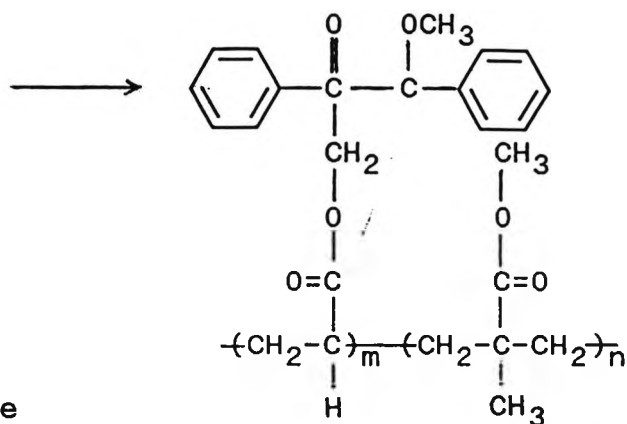
MB/MMA Copolymers
