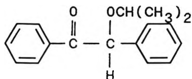
BIPE
