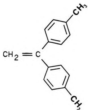
1,1-Ditolylethylene (DTE) 2,2,6,6-Tetramethylpiperidinoxyl Radical (T.M.P.O.)
