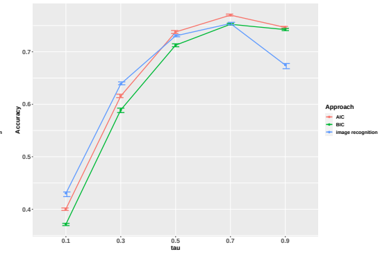
(d) n = 250
