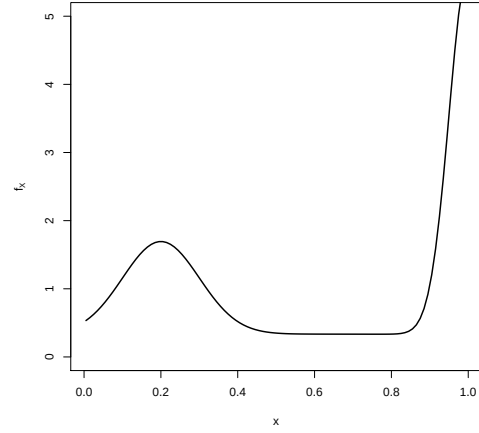
(b) f_X : Boundary challenge.
