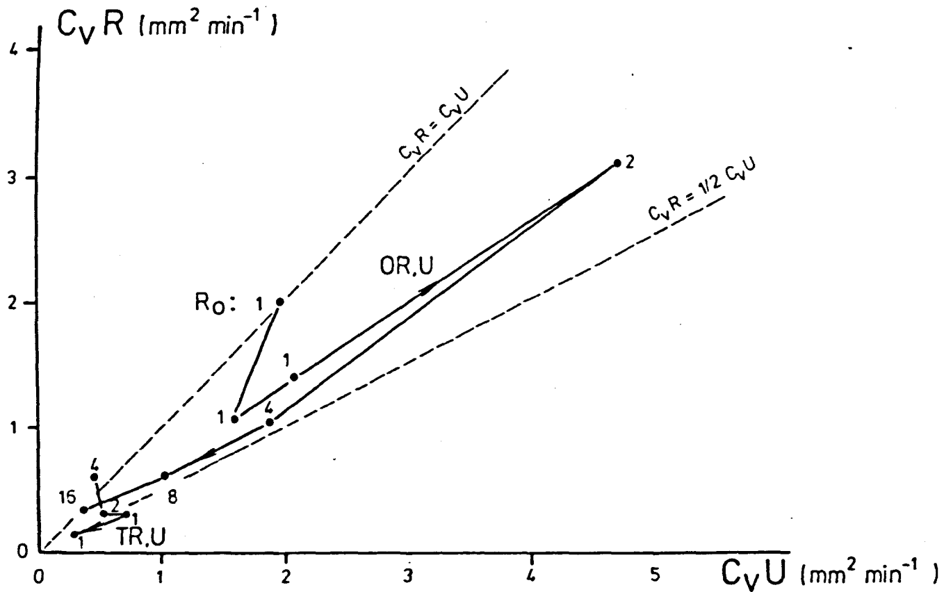
Figure 8.26 \frac{C_V R}{C_V U} : \frac{C_V U}{C_V U} : till HH(b) (Tests OR(2) , OU(2)V ; TR(2) , TU(2)).
