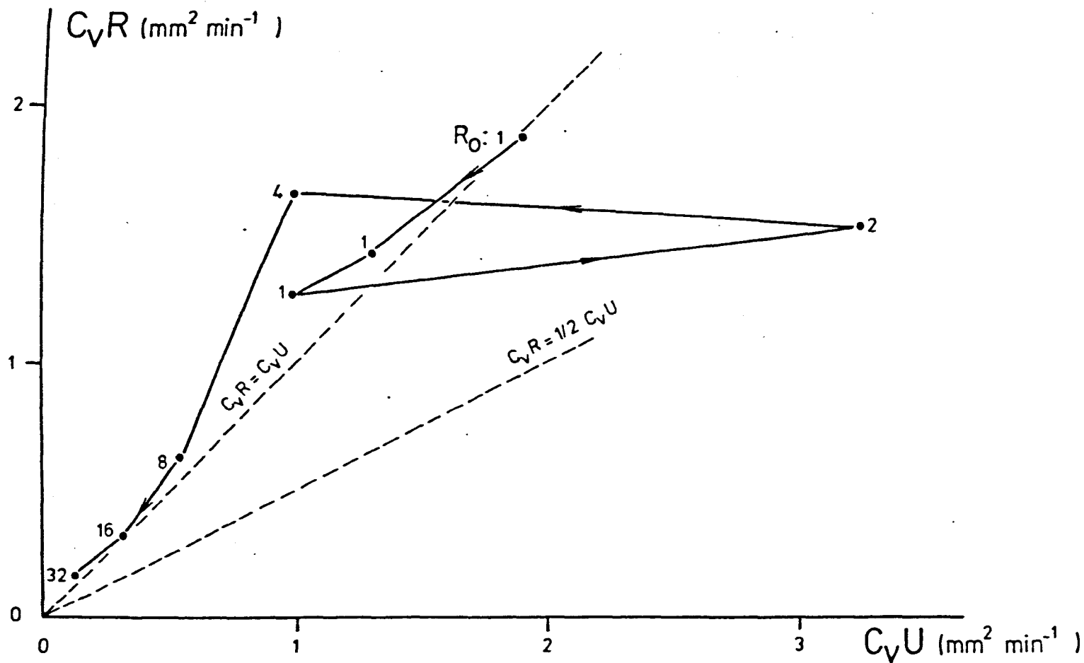
Figure 8.29 \frac{c}{v} R : \frac{c}{v} U : \text{till } w(d) (Tests OR(5), OU(5)V).
