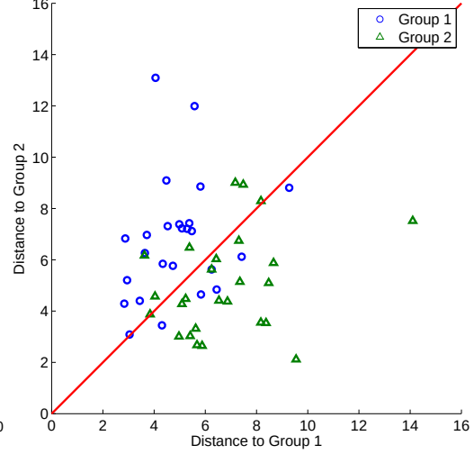
(d) SIMCA-D. p = 1250 , \frac{n_k}{p} = 0.02 .
