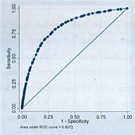
AUC = 0.8072 (b)
