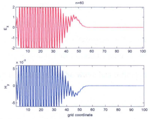
(d) Distorted Gaussian pulse at time step n = 60 .
