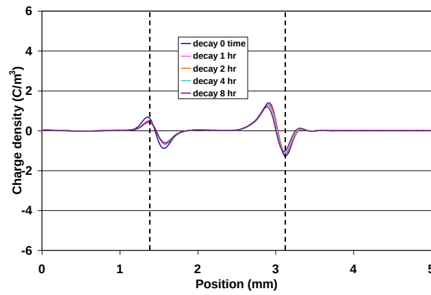
(d) Space charge decay
