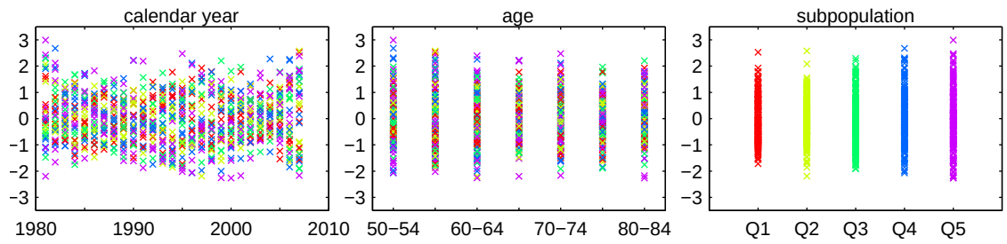
(D) Joint- \kappa : \log_n \mu_{xtg} = \alpha_x + \alpha_{xg} + (\beta_x + \beta_{xg}) \kappa_t
