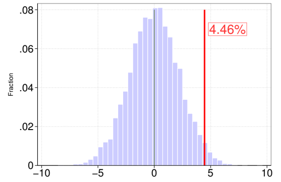
(d) \text{Distr}(\bar{Z}^{mom}) under H_0: \bar{Z}^{mom} = 0
