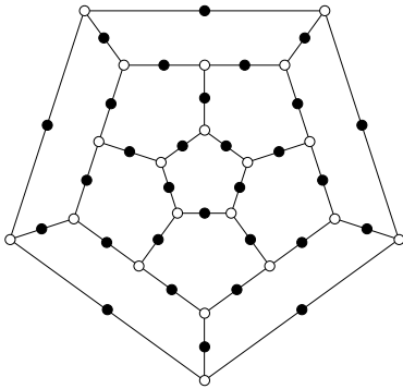
\Gamma(5) 5, 5, 5, 5, 5, 5, 5, 5, 5, 5
