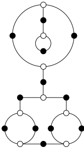
9, 5, 5, 2, 2, 1 ( \mathbb{Q} )
