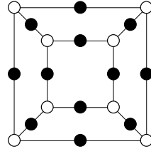
4, 4, 4, 4, 4, 4 ( \mathbb{Q} )
