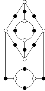
5, 5, 5, 5, 2, 2 ( \mathbb{Q} )
