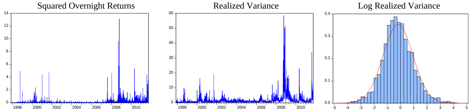
(b) S&P 500
