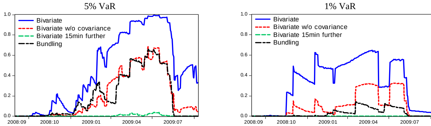
(b) S&P 500
