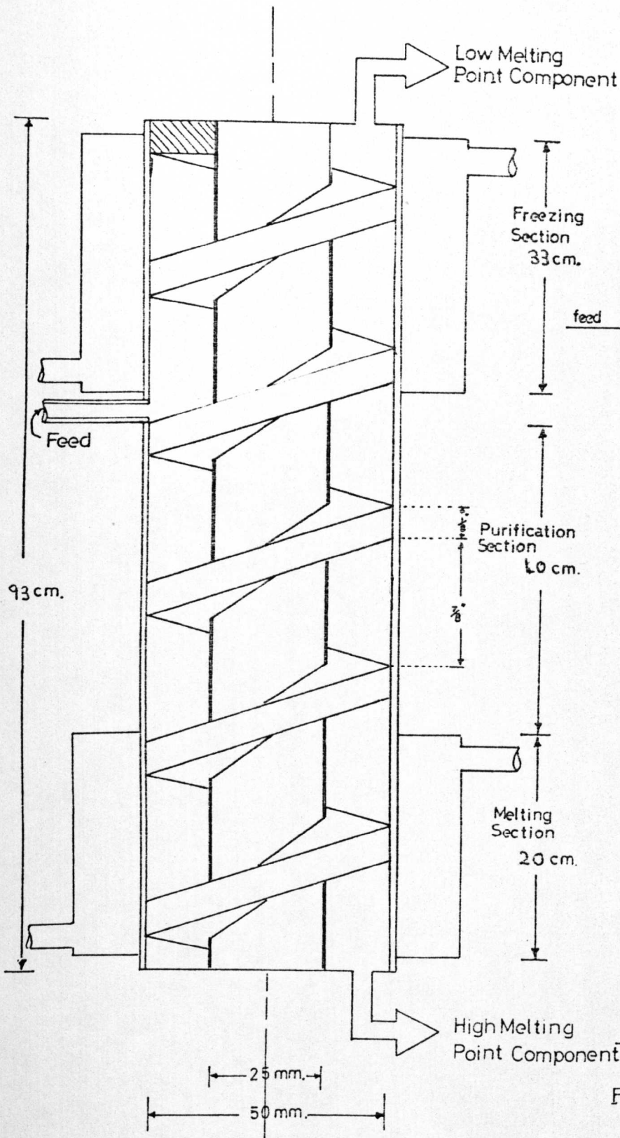
FIG.1. COLUMN CRYSTALLIZER
