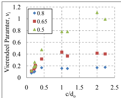
Figure 4: Typical values for ‘Vierendeel’ parameter
